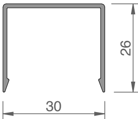
FWP00003 tapa perfil refuerzo
