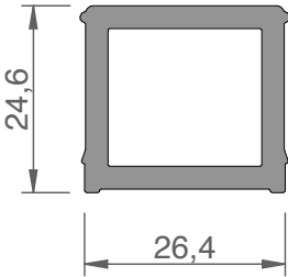
FWP00002 perfil refuerzo
