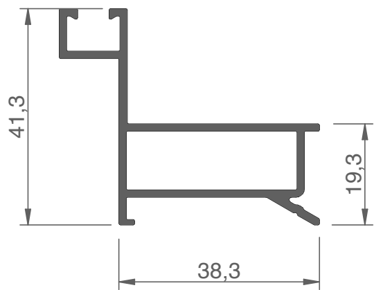
FWP20002 marco multicarri
