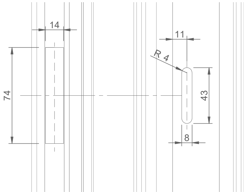
Mecanizado hoja principal
