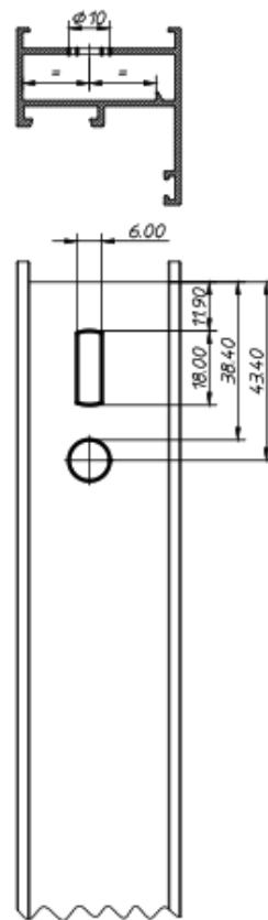
C Operación escuadra marco practicable
