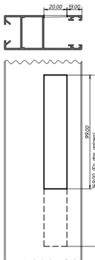
G Operación cierre embutido grande
