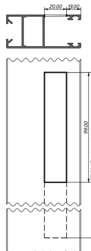
G Operación cierre embutido pequeño
