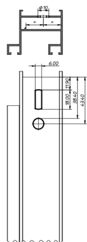
C Operación escuadra marco corredera
