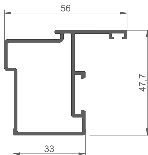
FWP10004 complemento cerradura
