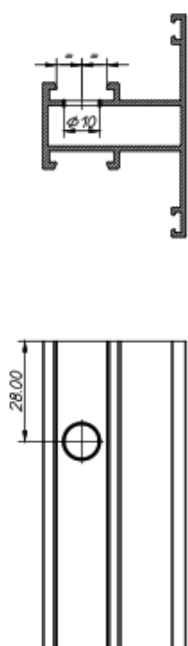
D Operación travesaño
