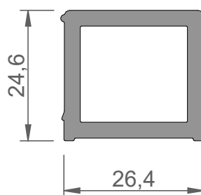
FWP00002 perfil refuerzo
