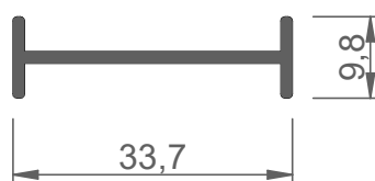
FWP00004 perfil unión
