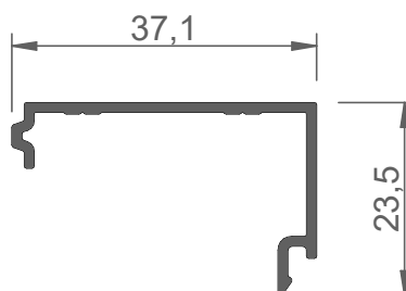
FWP00003 tapa perfil refuerzo
