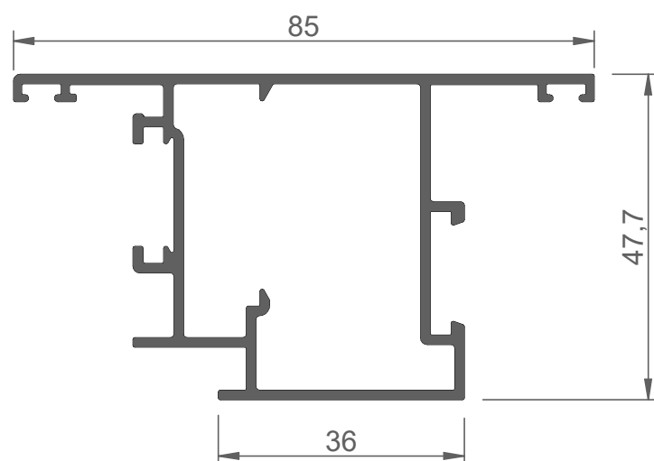
FWP10006 hoja apertura exterior
