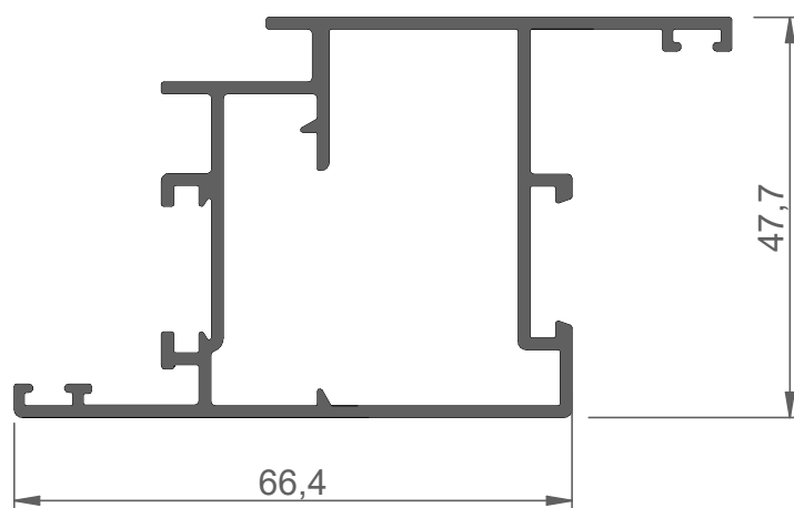
FWP00010 hoja apertura interior
