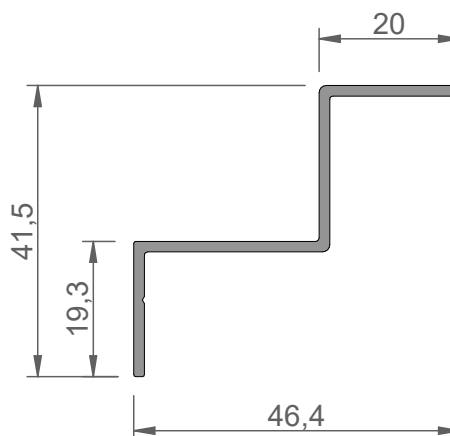
FWP00005 terminacion empotrado
