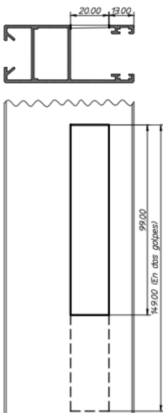
G Operación cierre embutido grande
