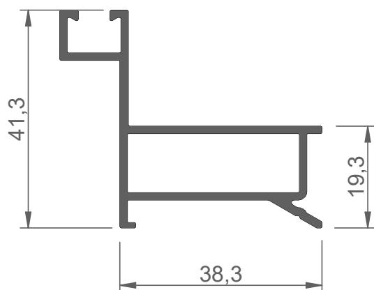
FWP20002 marco multicarril
