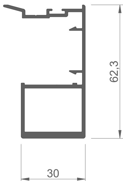
FWP20008 cruce hoja reforzado
