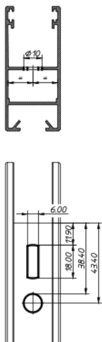
C Operación escuadra hoja corredera
