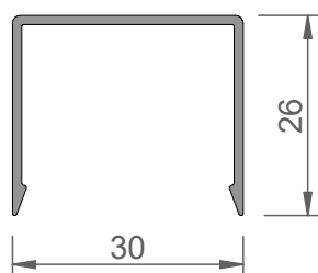
FWP00003 tapa refuerzo
