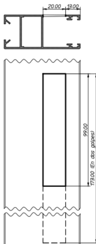
G Operación cierre embutido pequeño
